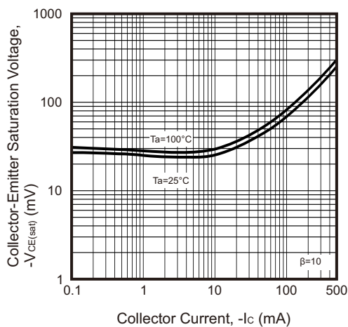
Fig.3 - V_{CEsat} - I_C
