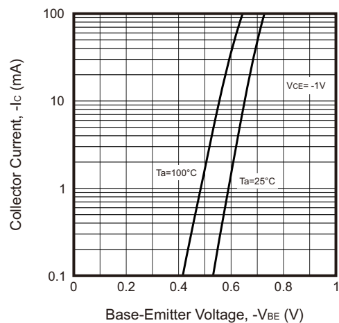
Fig.4 - V_{BE} - I_C
